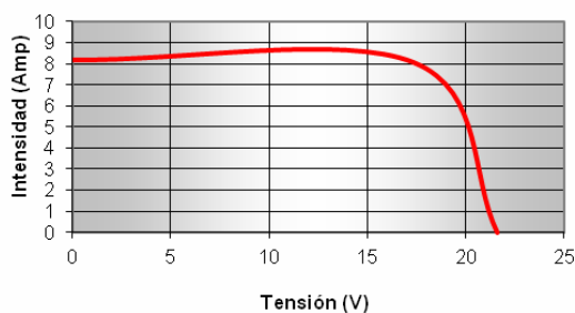
Curva I-V (1.000W/m 2 , AM 1.5, 25°C)
